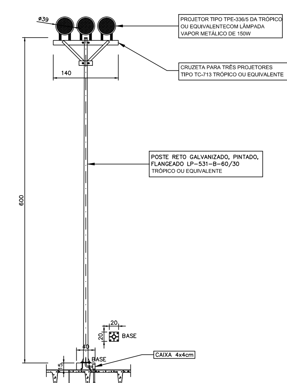
D-9 DETALHE 9- PROJETORES MEM POSTE PARA ILUMINAÇÃO DA QUADRA ESCALA 1:50
