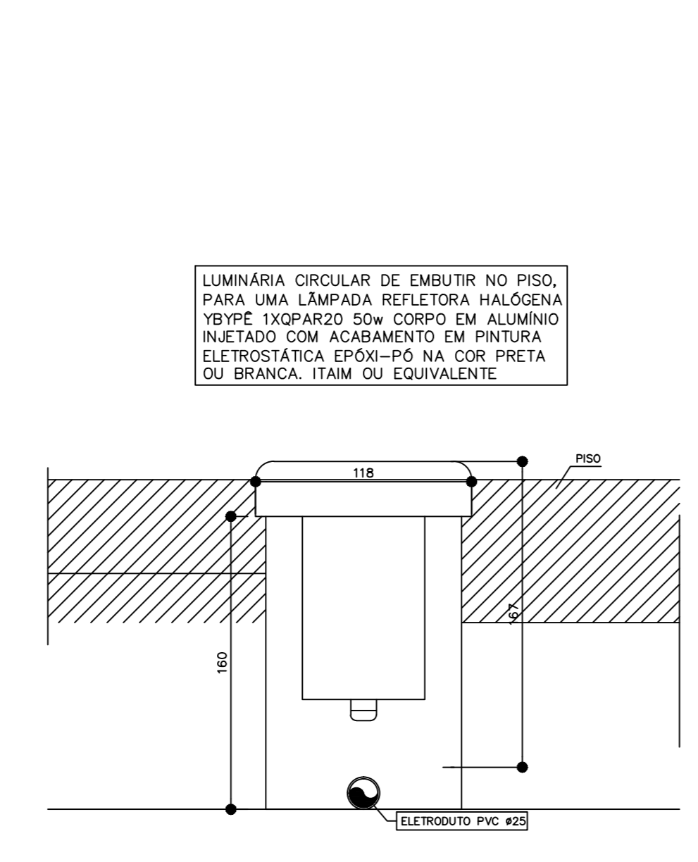
D-11 DETALHE 11- LUMINARIA NO PISO DO DECK ESCALA 1:20
